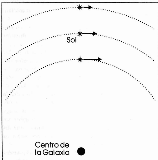
Diagrama con la representación de los movimientos de las estrellas cerca del Sol. Las estrellas más cercanas al centro de la Galaxia que el Sol se mueven más rápido que éste, mientras que las más externas lo hacen más lentamente.
