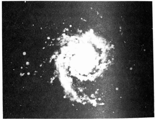
Fotografía de una galaxia espiral en la constelación de Piscis. El plano de esta galaxia es perpendicular a la línea de la visual.
