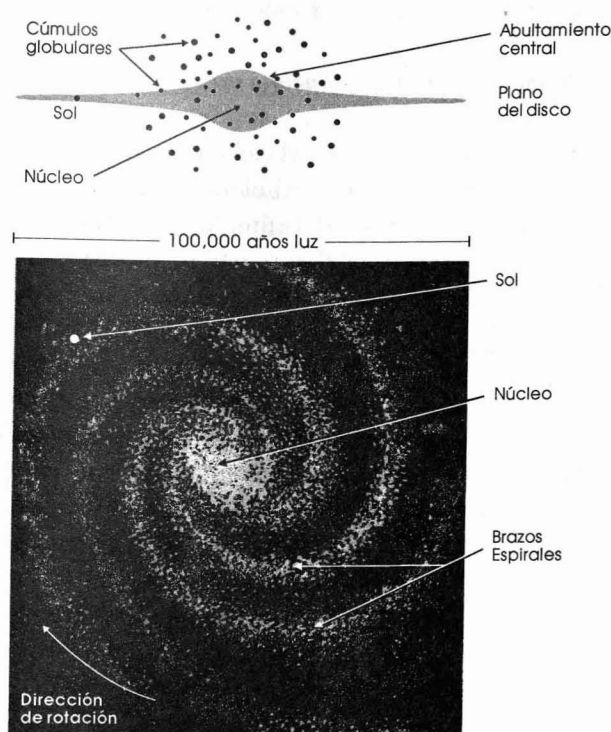
Diagrama de la estructura de la Galaxia.
