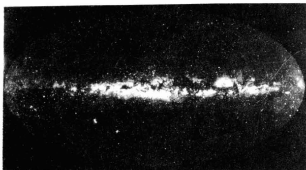
Mosaico fotográfico del cielo nocturno. La figura está contruida de manera que la Vía Láctea aparezca en el ecuador.
