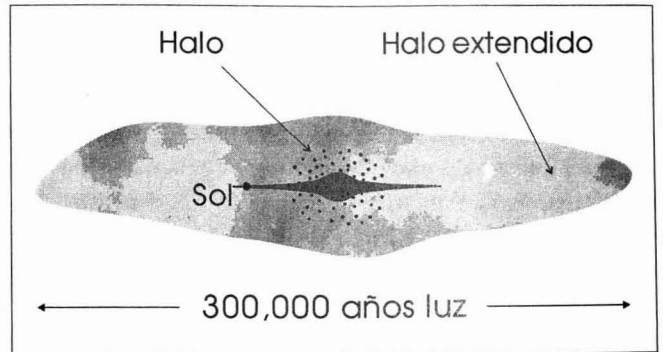
Diagrama del halo oscuro y extendido de la Galaxia. Se ilustra la forma y escala del halo extendido cuya presencia se deriva de los movimientos de rotación de las estrellas.
